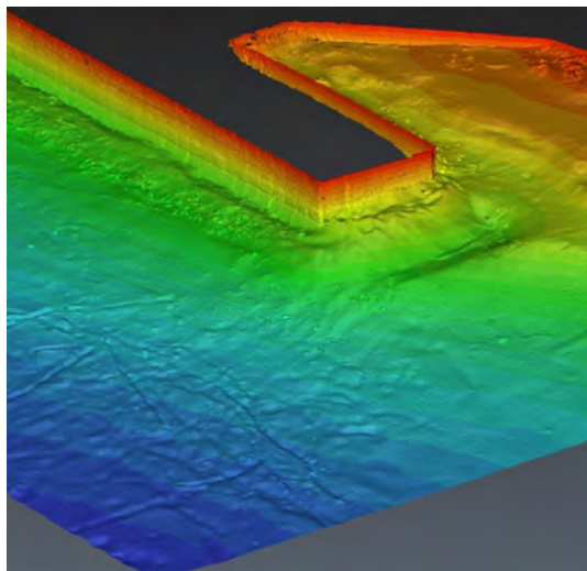
Τρισδιάστατη μορφολογική απεικόνιση του πυθμένα και των κρητιδώματων λιμένα
