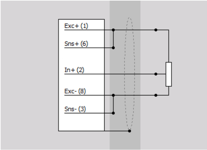
Potentiometer
